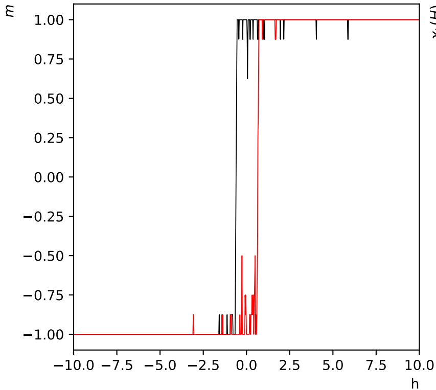
Hystérésis de l'aimantation réseau de taille L=4 - h=10 à T=2.0
